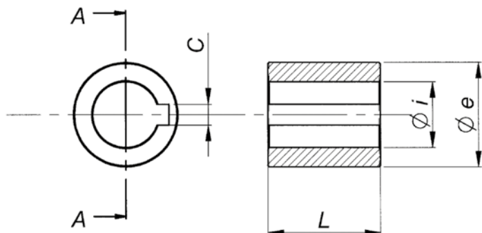
SEZ.: A-A
