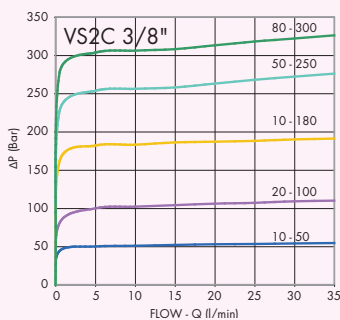
PRESSIONE/PORTATA PRESSURE/FLOW
