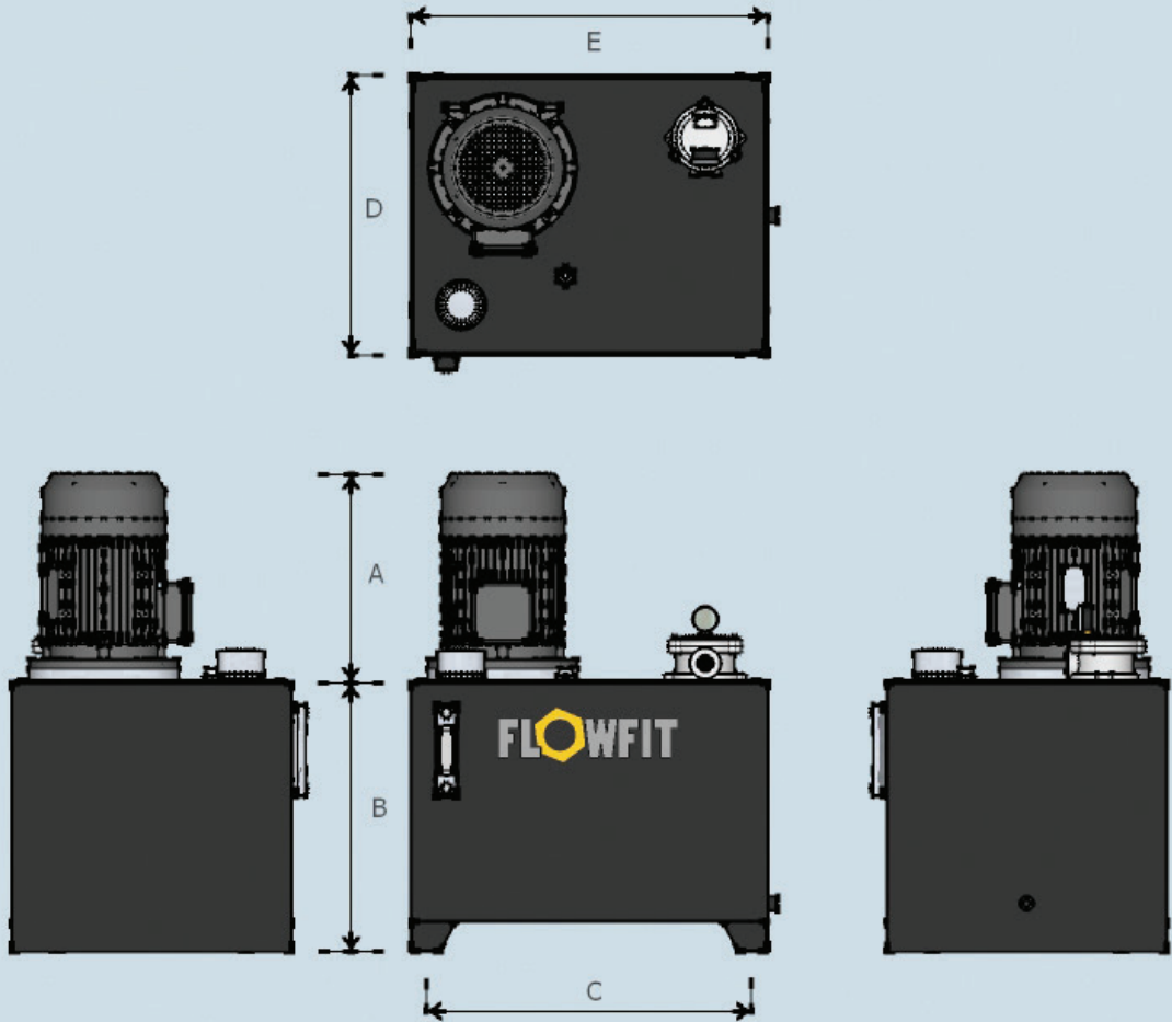
HF 500 Dimensions
