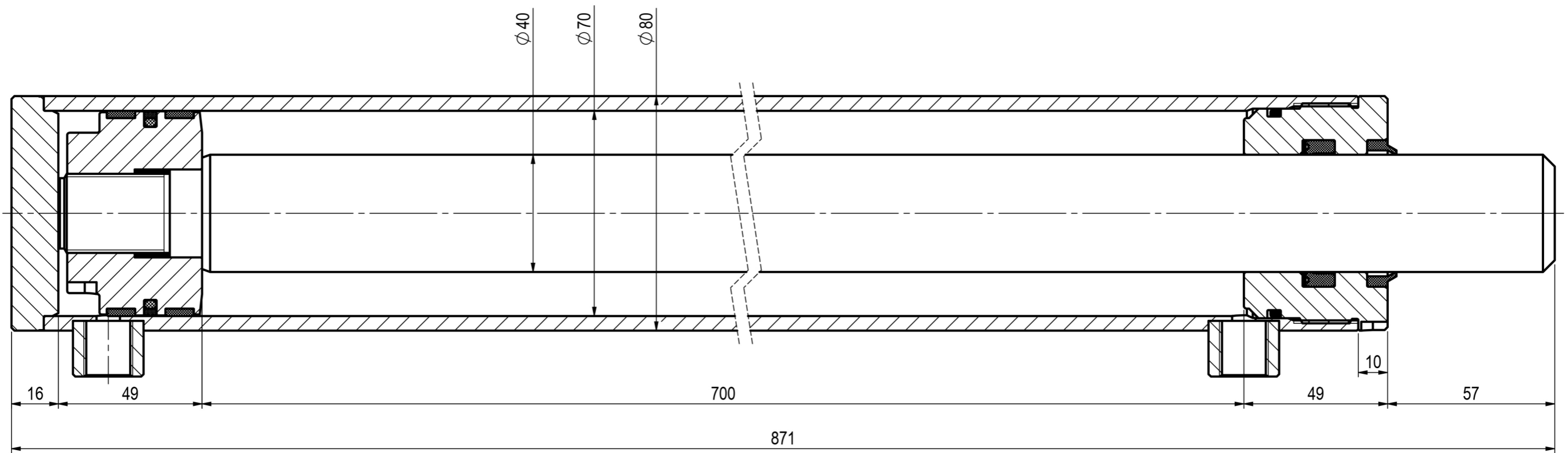
SECCIÓN A-A
