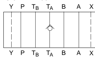
DGMDC-5N-X-T*-30
