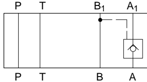
DGMPC-5-BA*-30
