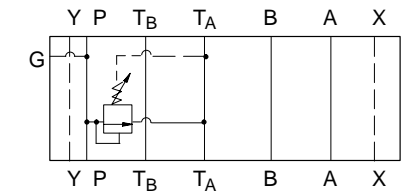
DGMC-5N-PT-**-30
