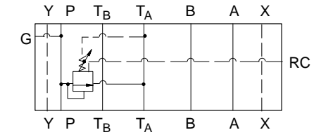
DGMC-5N-PT-**-RC-**-30
