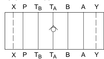
DGMDC-5P-X-T*-30
