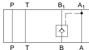
DGMPC-5-AB*-BA*-30
