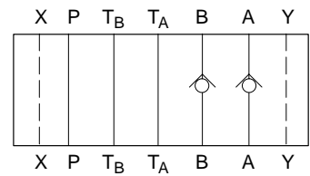
DGMDC-5P-Y-A*-B*-30
