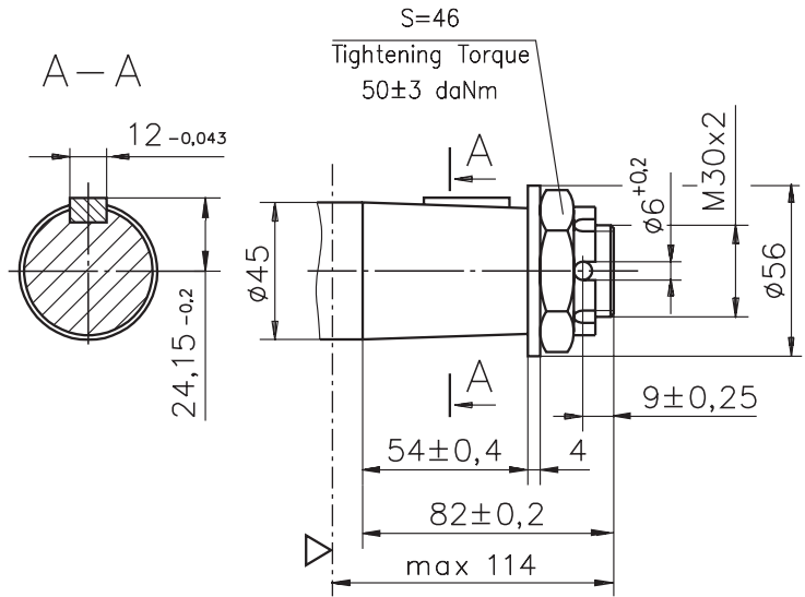
K -tapered 1:10, Parallel key B12x8x28 DIN 6885 Max. Torque 210,7 daNm
