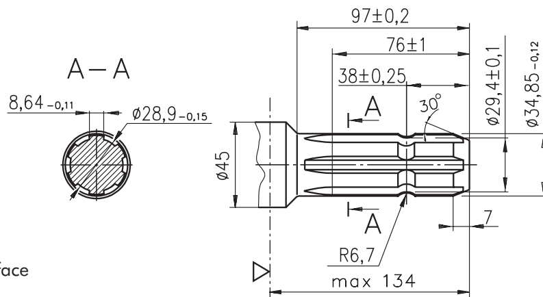
SL - \phi 34,85 p.t.o. DIN 9611 Form 1 Max. Torque 77 daNm
