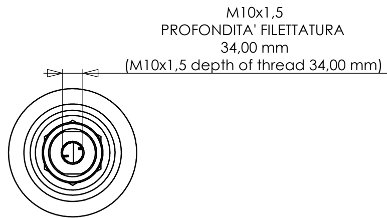
VISTA PARZIALE (Partial view)
