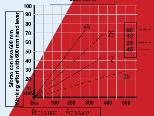
Diagramma prove di carico Load curve
